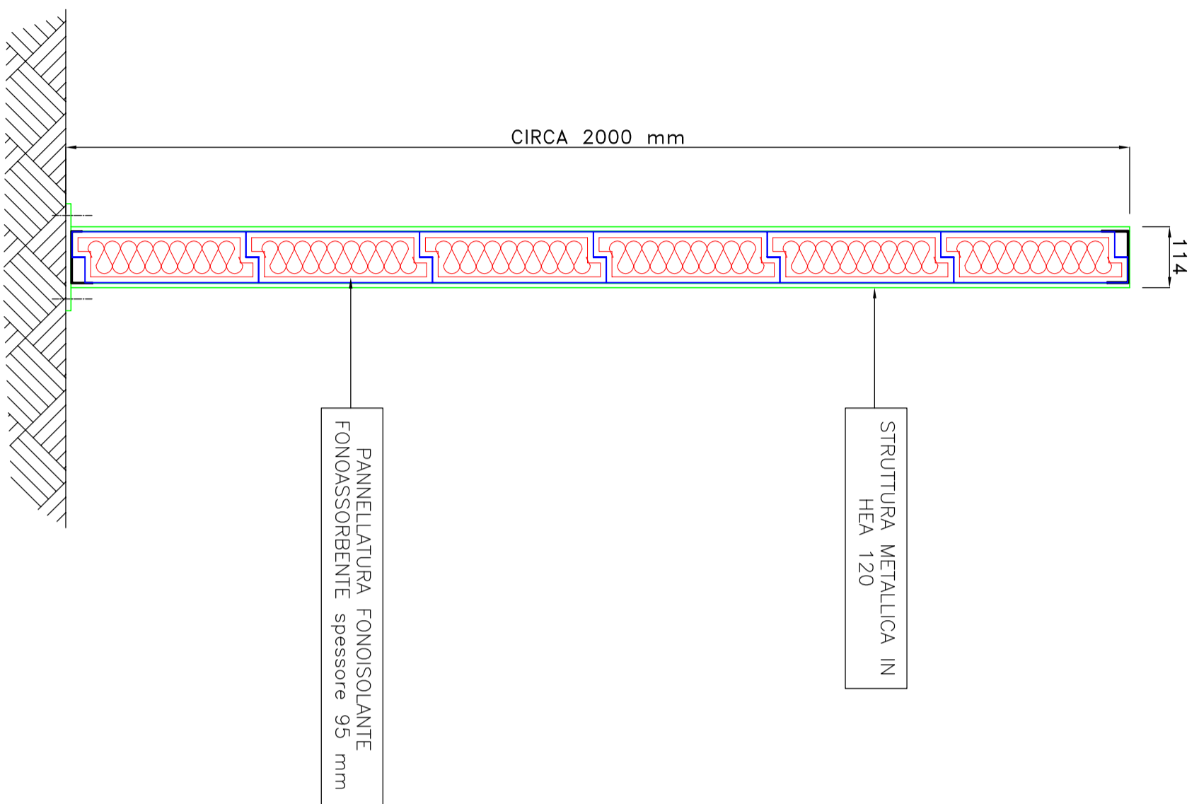
SEZIONE X-X BARRIERA sp.95 mm
