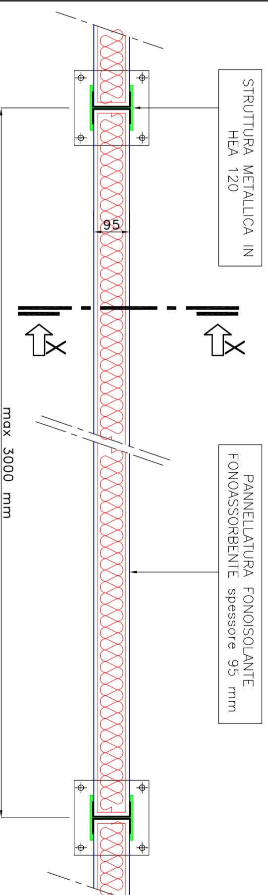
PIANTA BARRIERA sp.95 mm
